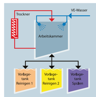
Schematischer Prozessablauf
